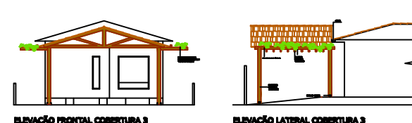
ELEVAÇÃO FRONTAL COBERTURA 3
