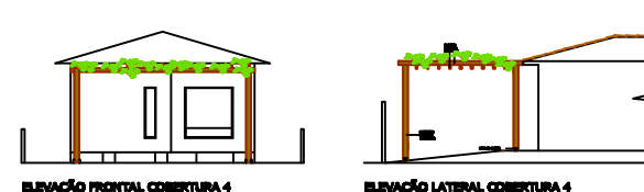
ELEVAÇÃO FRONTAL COBERTURA 4
