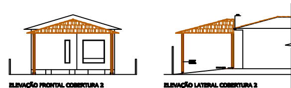
ELEVAÇÃO FRONTAL COBERTURA 2
