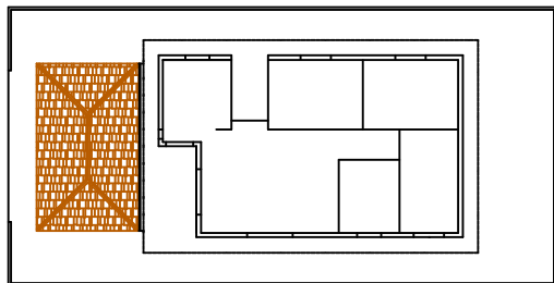
PLANTA COBERTURA 1
