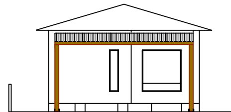
ELEVAÇÃO FRONTAL
