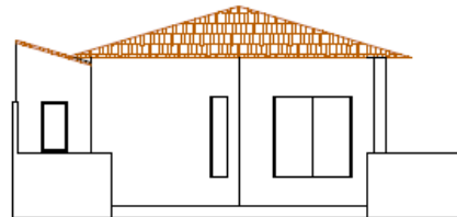
EDÍCULA 2 - ELEVÇÃO FRONTAL
