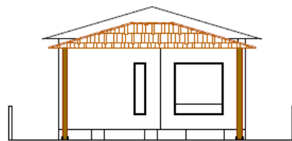
ELEVAÇÃO FRONTAL
