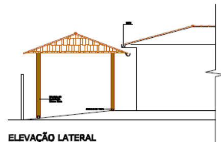
ELEVAÇÃO LATERAL
