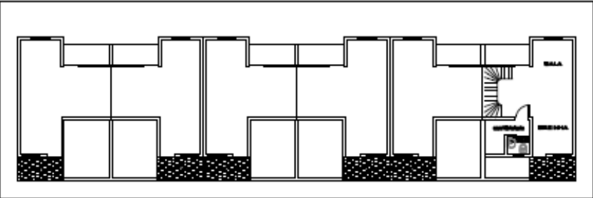
TÉRREO
