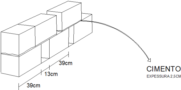
DETALHAMENTO DOS TIJOLOS ESPAÇADOS
