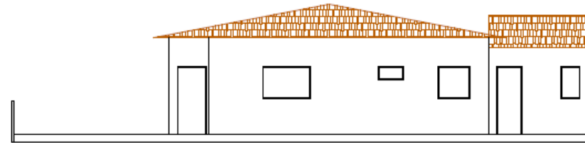
EDÍCULA 1 - ELEVÇÃO LATERAL
