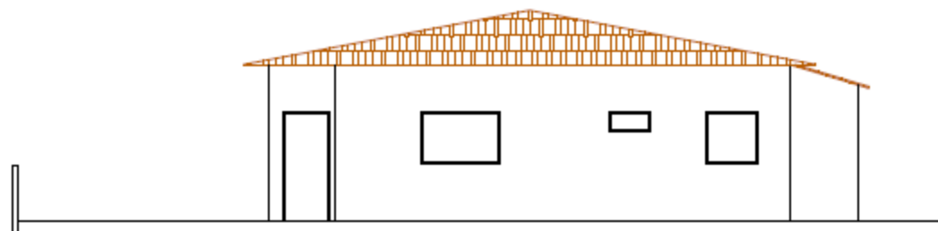
EDÍCULA 6 - ELEVÇÃO LATERAL
