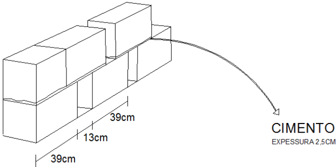
DETALHAMENTO DOS TIJOLOS ESPAÇADOS
