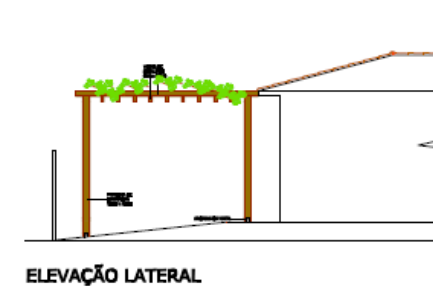
ELEVAÇÃO LATERAL
