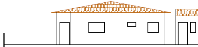
EDÍCULA 2 - ELEVÇÃO LATERAL
